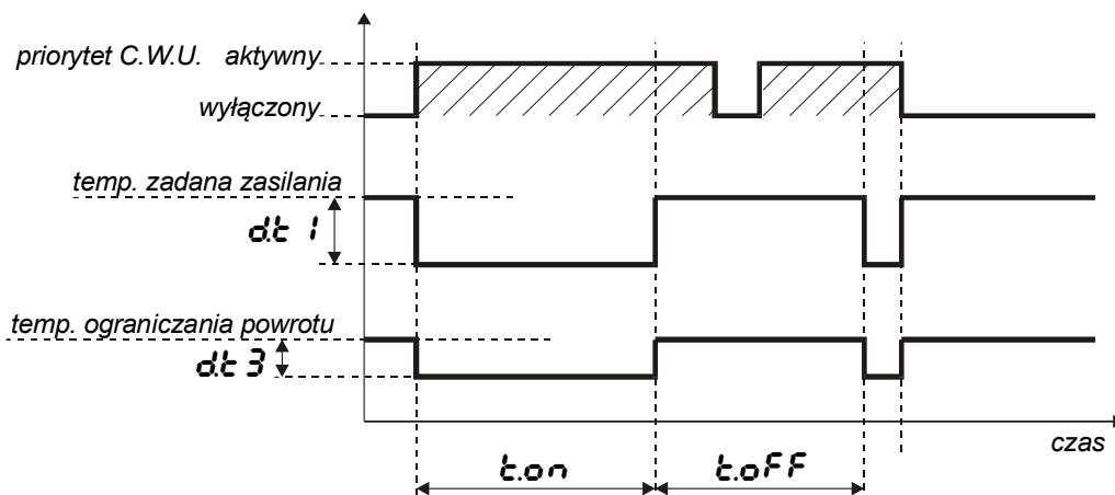
Rys. 21. Działanie priorytetu C.W.U. dla trójstawnego napędu zaworu.
