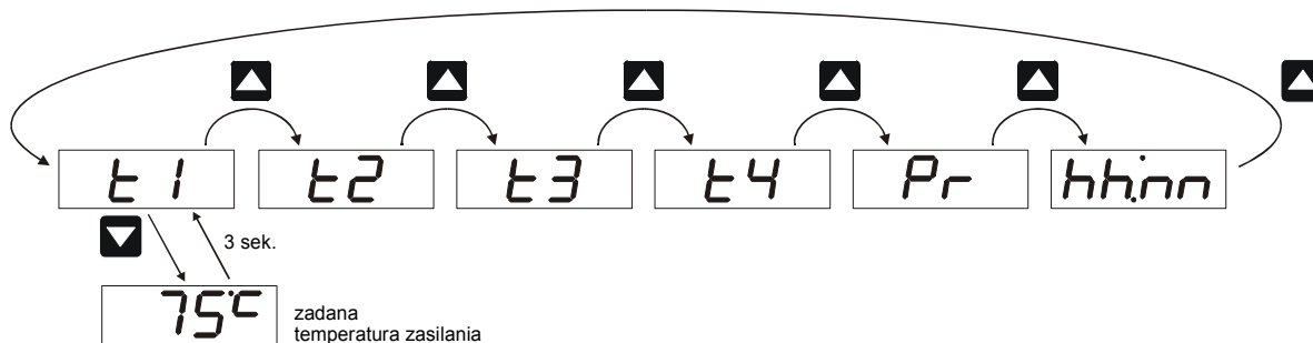
Rys. 17. Sposób odczytania wartości zadanej temperatury zasilania.
