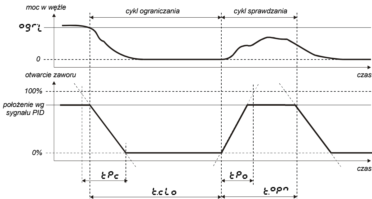
Rys. 30. Ograniczanie mocy minimalnej.
