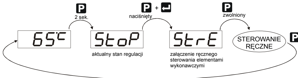
Rys. 15. Sterowanie ręczne.
