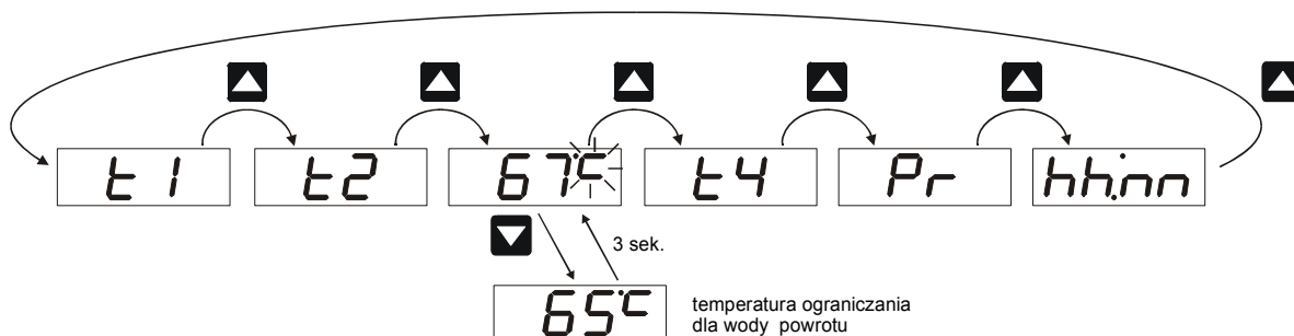
Rys. 19. Sygnalizacja aktywności ograniczania temperatury dla wody powrotu.
