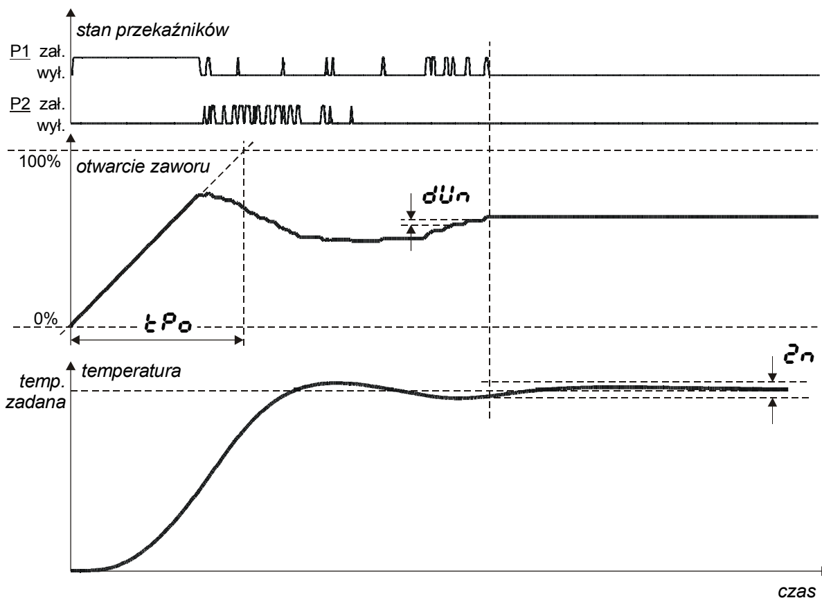
Rys. 12. Algorytm trójstawny krokowy PID.
