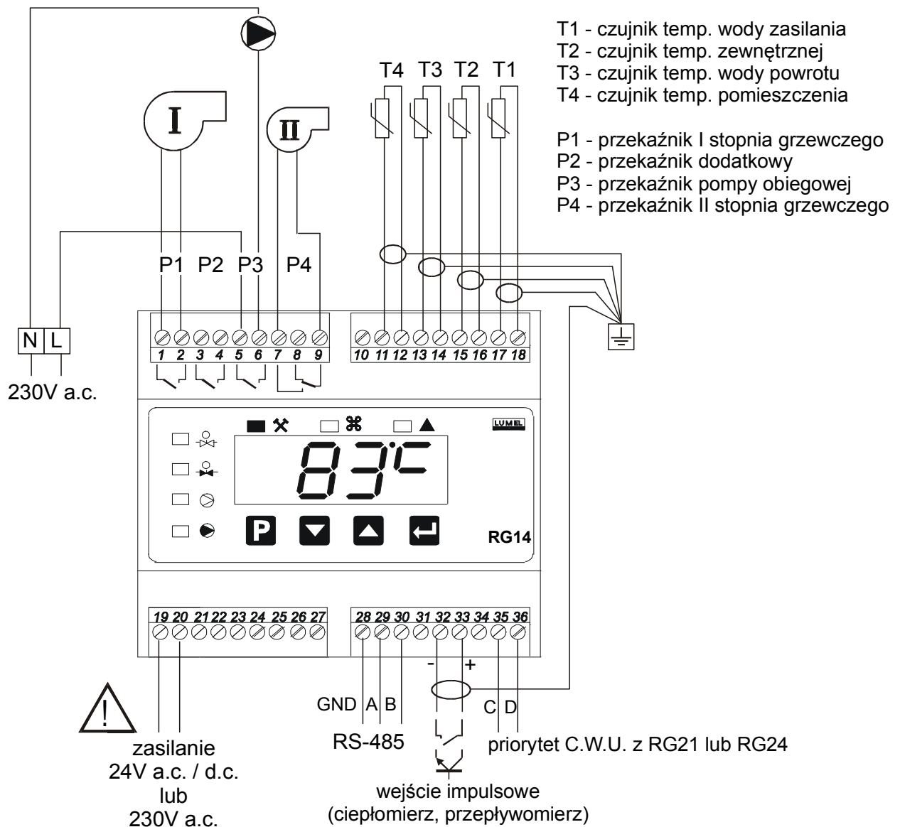
Rys. 6. Połączenia zewnętrzne regulatora do sterowania węzłem z kotłem dwustopniowym i pompą obiegową.
